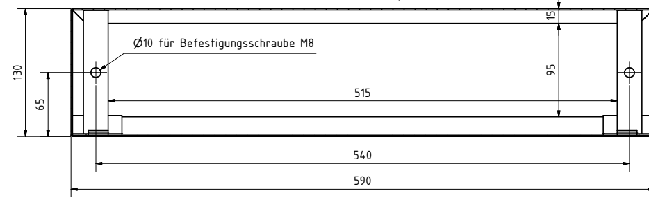
A-A ( 1 : 2,5 )
